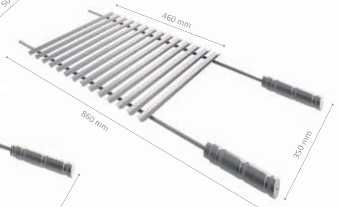
440 • GRELHA INOX PROFISSIONAL 7 896621 00440 3
